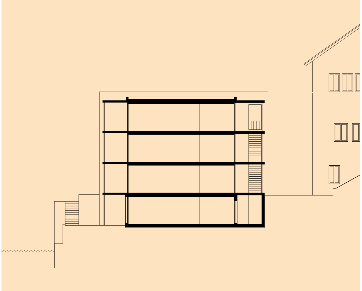
QUERSCHNITT
