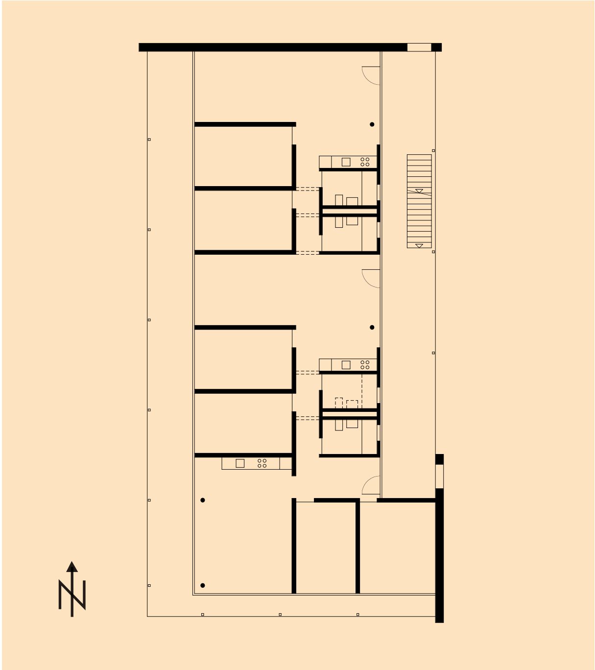
GRUNDRISSE EG/0G
